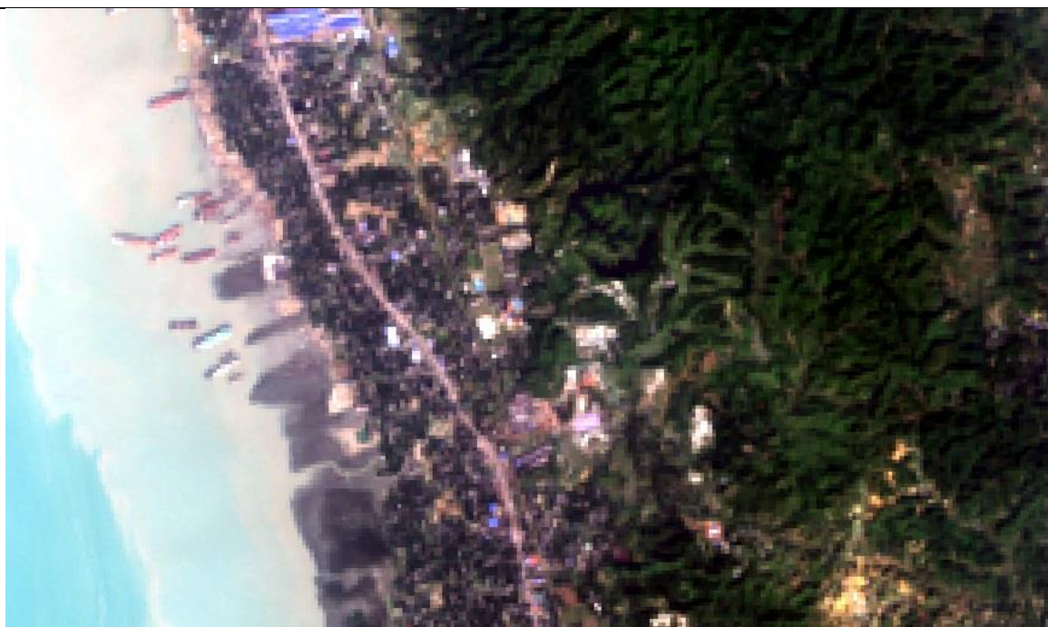
Image satellitaire prise par le capteur «Landsat 8»
